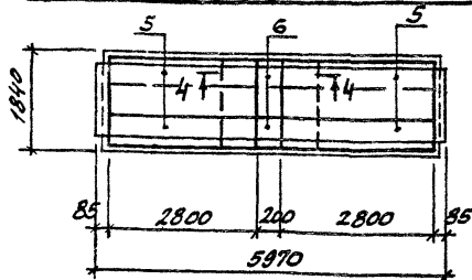
ПЛАН РАСКЛАДКИ УГЛОВЫХ СЕТОК ДЛИНОЙ 2,85м ПРИ СТЫКАХ В ПРОДОЛЬНОМ И ПОПЕРЕЧНОМ НАПРАВ- ЛЕНИЯХ ДЛЯ ПИ-12, ПИ-15
